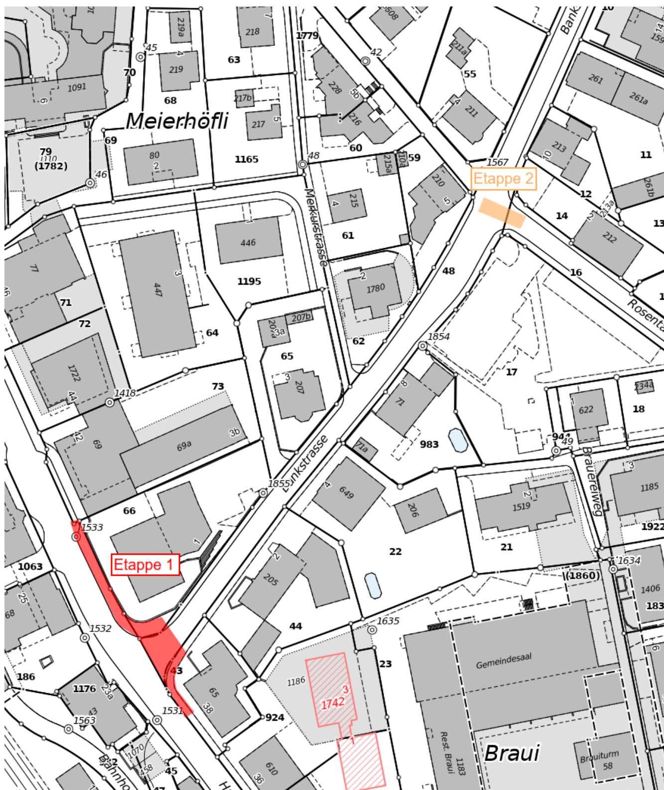
Übersicht Werkleitungserneuerung Bankstrasse, Hochdorf
